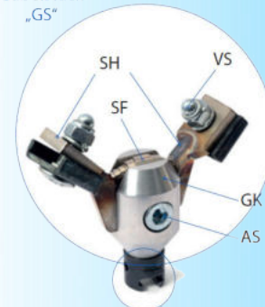
Gabelstück „GS“
